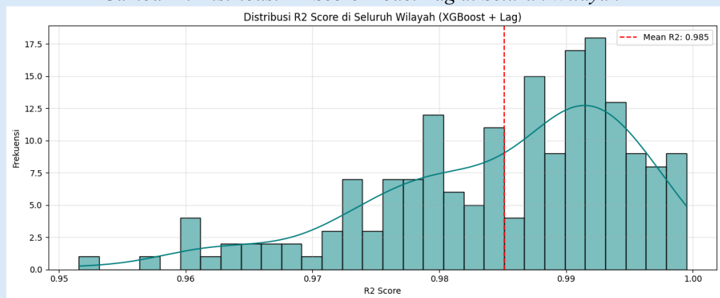
Gambar 1. Distribusi R2 Score Model Lag di Seluruh Wilayah
